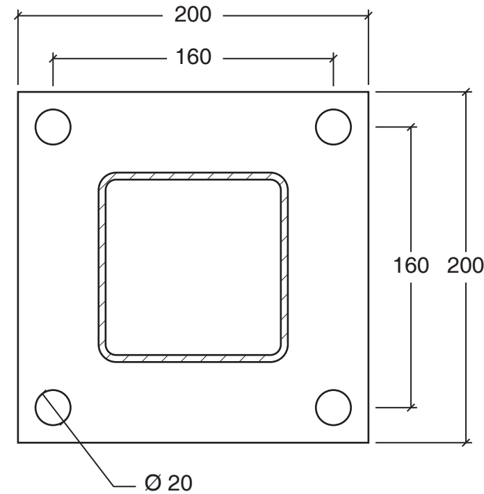
DETAIL A-A SCALE 1:3
